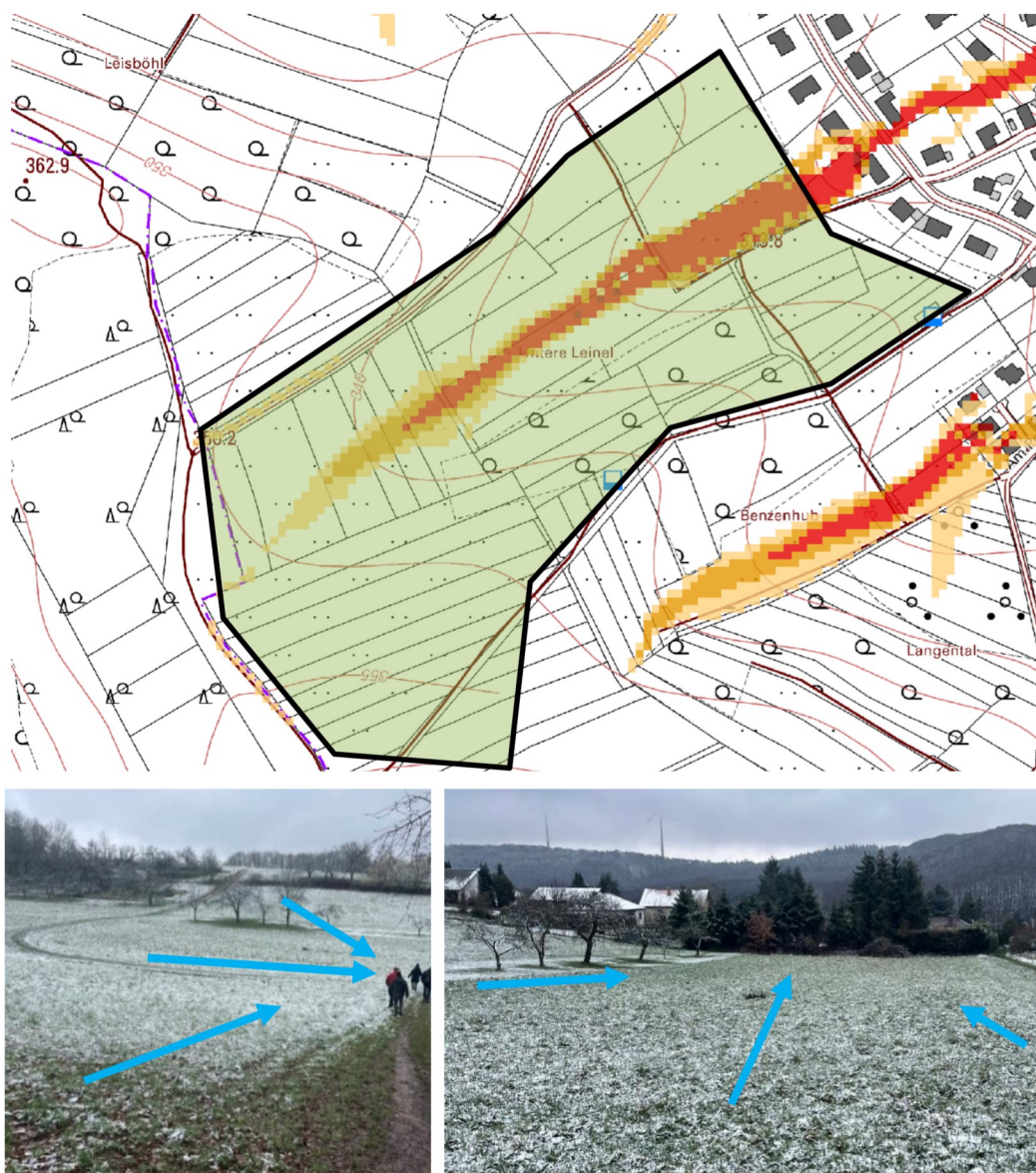
Abbildung 13: "Untere Leinel", Außeneinzugsgebiet (grün) und Fließwege (blau)
