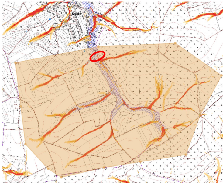
Abbildung 18: Außeneinzugsgebiet am südlichen Ortsrand/Hauptstraße
