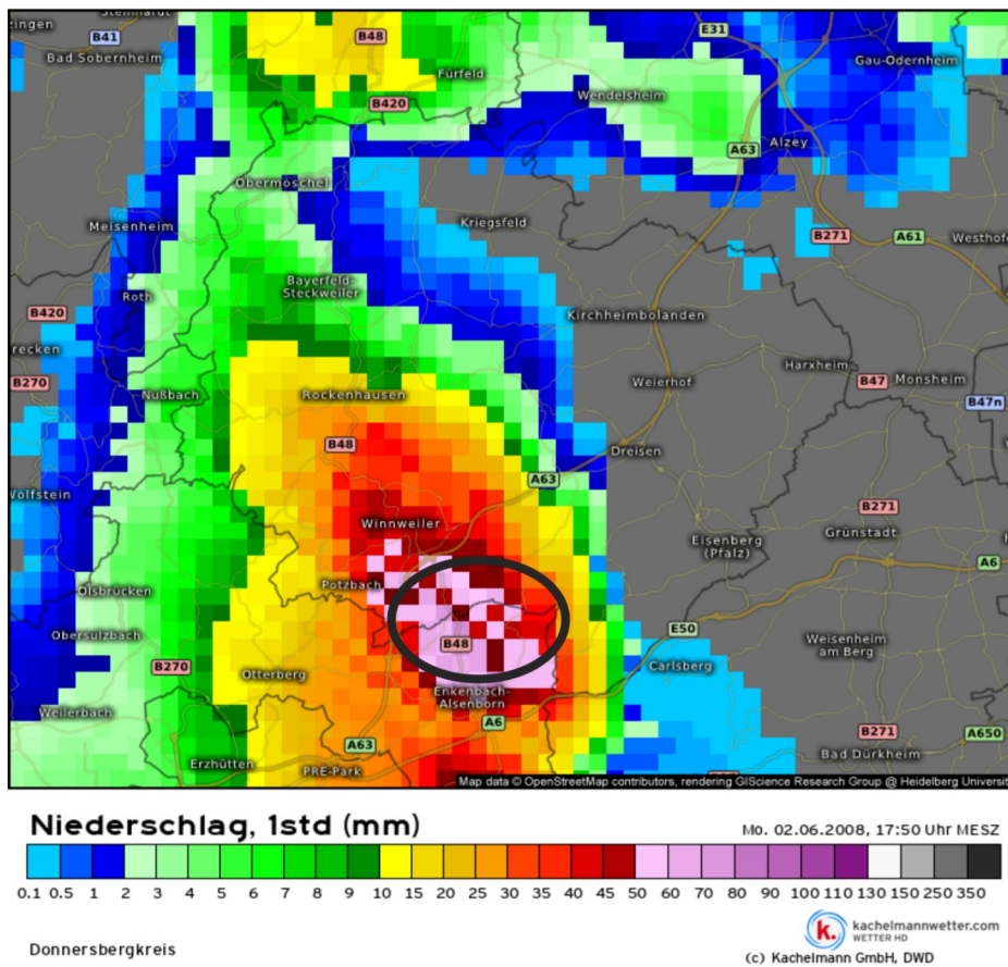
Abbildung 3: Regenradar Donnersbergkreis vom 02.06.2008 (Kachelmannwetter.com)
