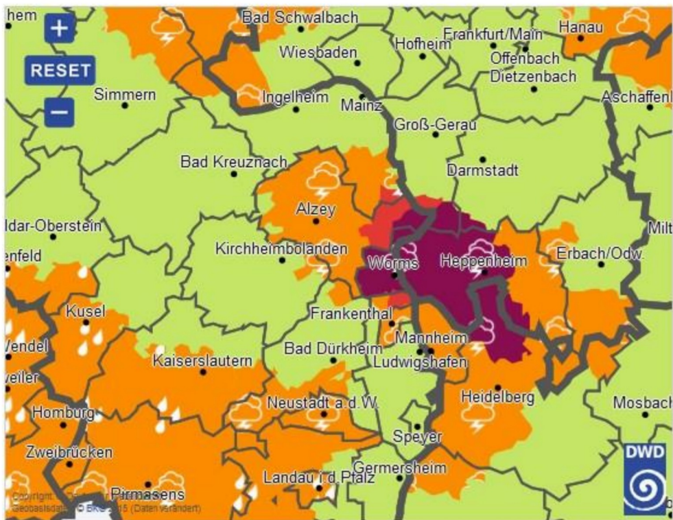
Abbildung 62: Warnkarte des DWD (Beispiel)
